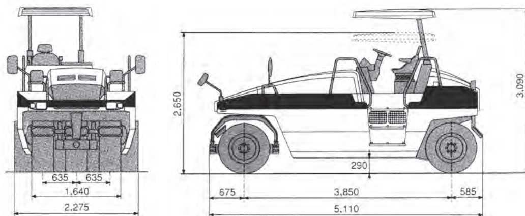
主要寸法図
