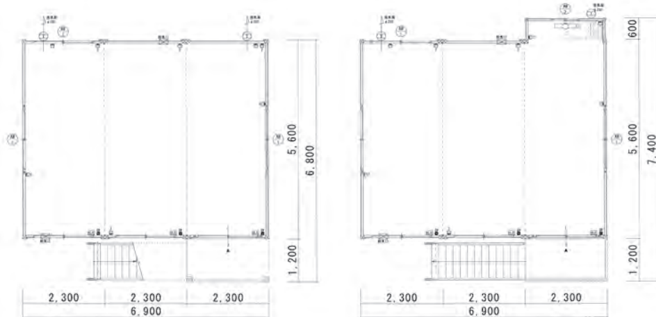
例：3連棟2階建てキッチン付平面図
